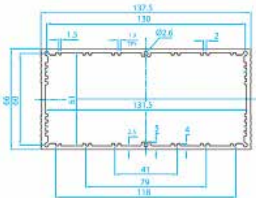
Cut-out to DIN 43700 68x138
