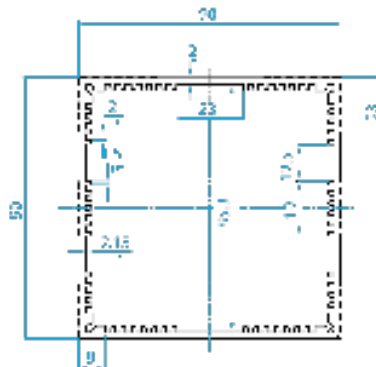
Cut-out to DIN 43700 92x92
